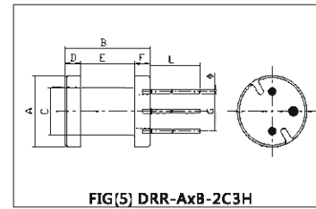
FIG(5) DRR-AxB-2C3H
