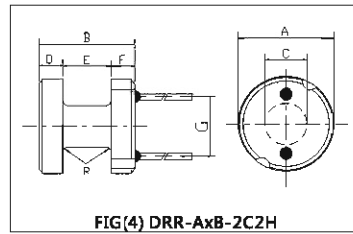
FIG(4) DRR-AxB-2C2H
