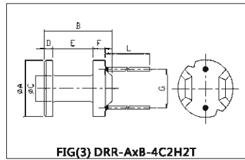
FIG(3) DRR-AxB-4C2H2T
